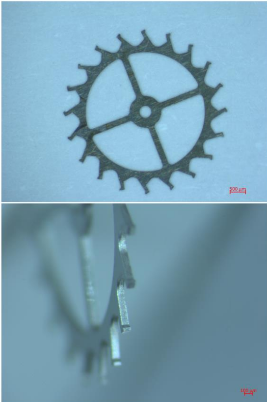
Figure 3 : Roue d'échappement.
